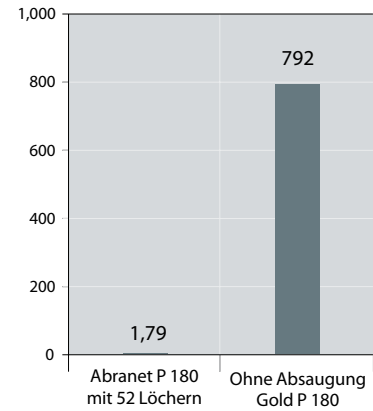
Staub auf den Oberflächen der Umgebung (g/kg NTP)
