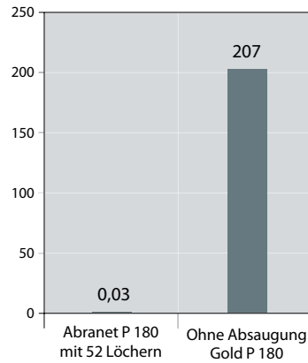
Staubgehalt der Luft pro kg geschliffenen materials (g/kg NTP)
